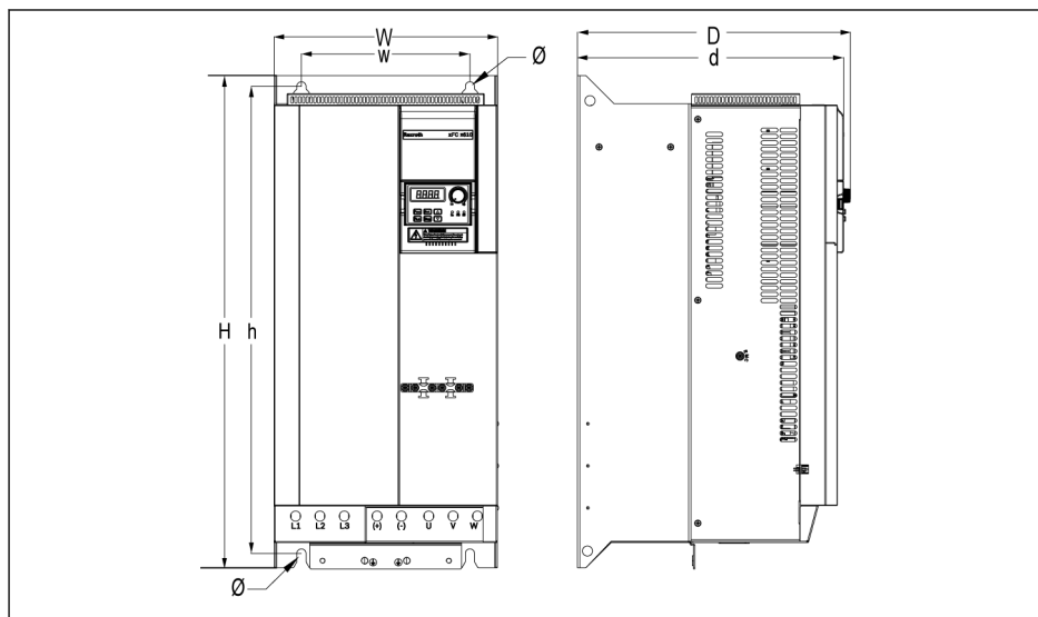
Рис. 7-5: Размерный чертёж VFC 5610 45K0...55K0
