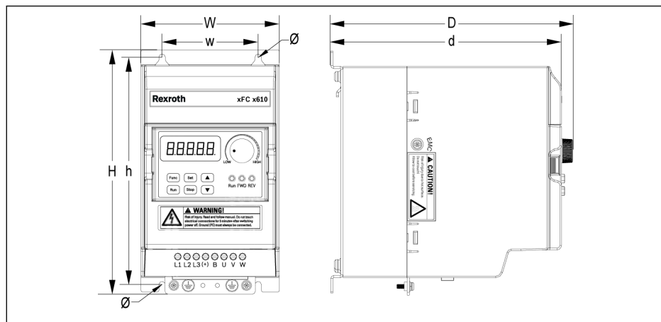
Рис. 7-2: Размерный чертёж VFC x610 OK40...4K00
