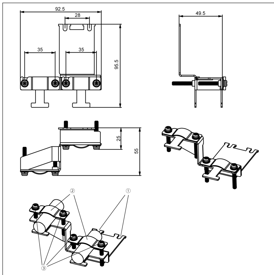
Рис. 15-30: Присоединение экранированного кабеля с принадлежностями для 5K50...22K0 (FEAM03.2-002-NN-NNN)
