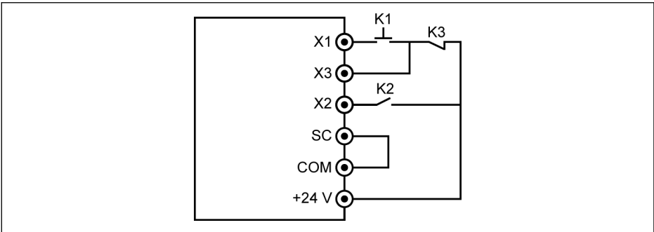
Рис. 12-39: 3-проводной режим управления 1
