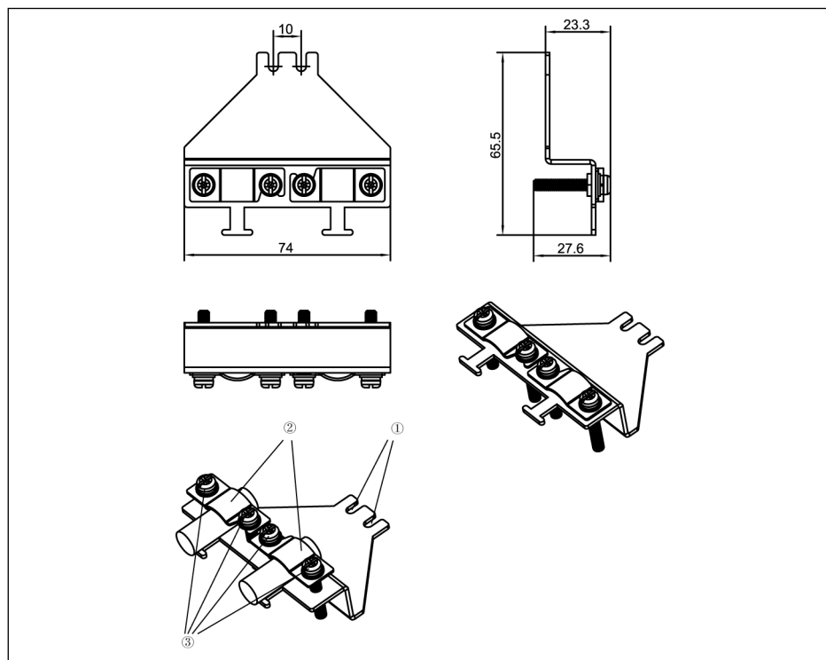
Рис. 15-29: Присоединение экранированного кабеля с принадлежностями для OK40...4K00 (FEAM03.2-001-NN-NNN)
