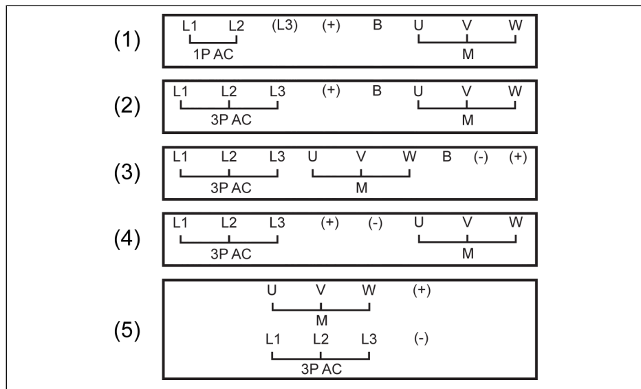
Рисунок клемм питания
