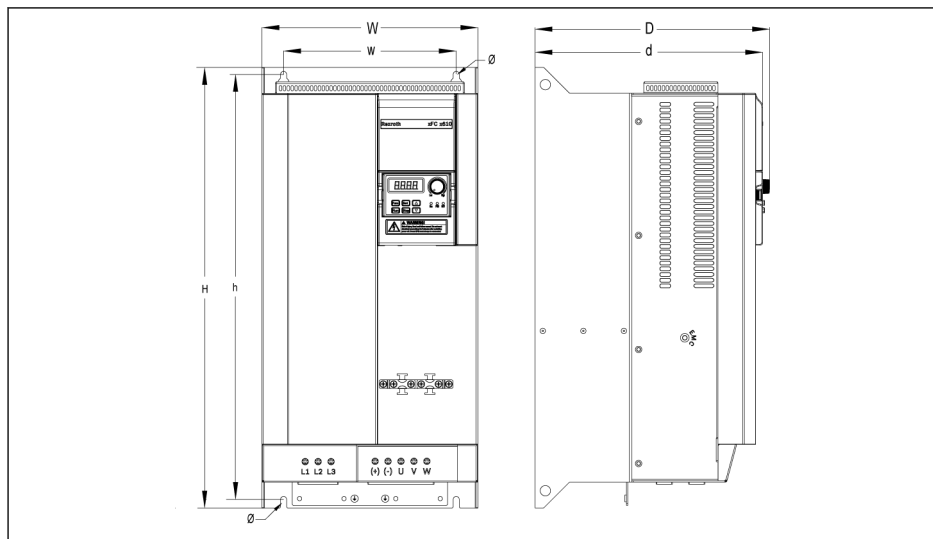
Рис. 7-4: Размерный чертёж VFC 5610 30K0...37K0
