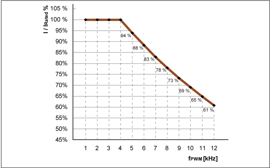
Рис. 6-5: Снижение характеристик и несущая частота для моделей 30K0...90K0 (нормальный и интенсивный режимы)
