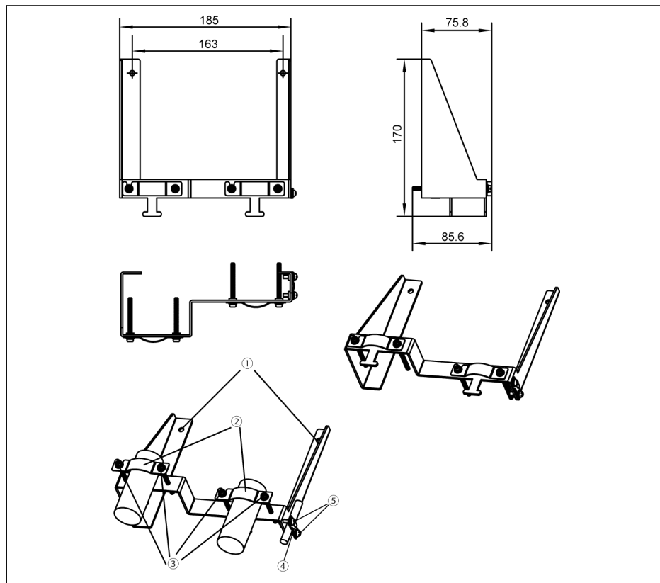
Рис. 15-31: Присоединение экранированного кабеля с принадлежностями для 30K0...37K0 (FEAM03.2-003-NN-NNN)
