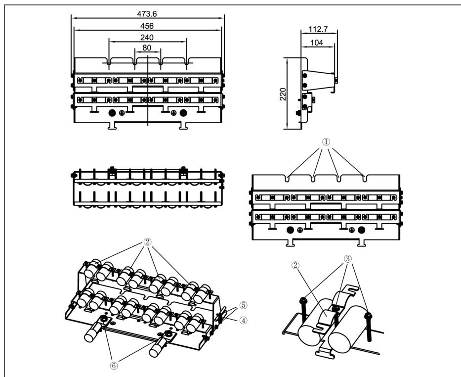
Рис. 15-34: Присоединение экранированного кабеля с принадлежностями для 160K...185K (FEAM03.2-006-NN-NNNN)
