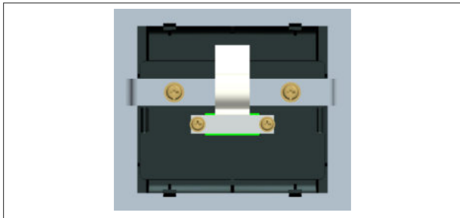
Рис. 15-5: Присоедините и зафиксируйте кабель (вид сзади)
