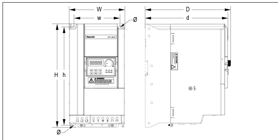
Рис. 7-3: Размерный чертёж VFC x610 5K50...22K0
