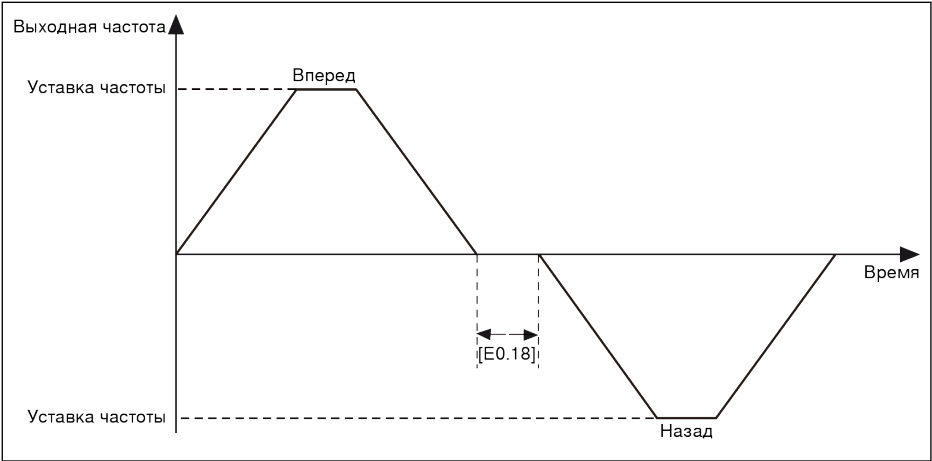
Рис. 12-27: Время задержки смены направления
