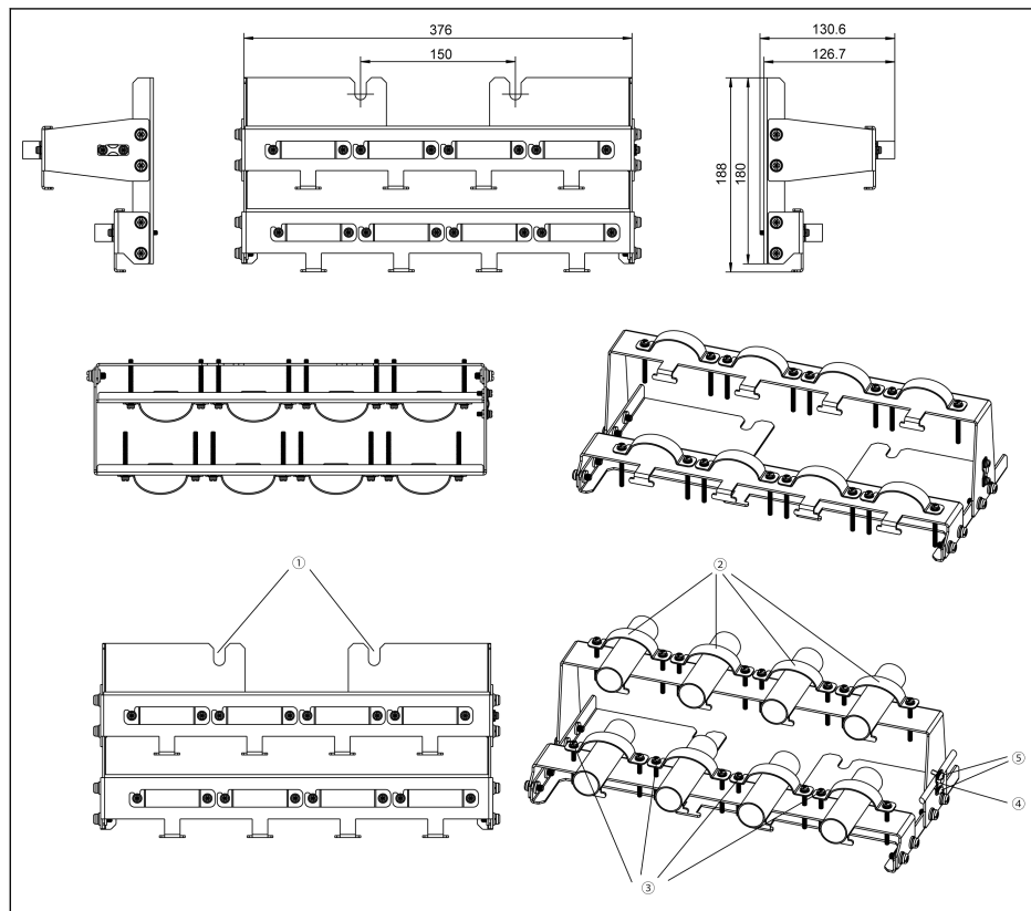
Рис. 15-33: Присоединение экранированного кабеля с принадлежностями для 110K...132K (FEAM03.2-005-NN-NNNN)
