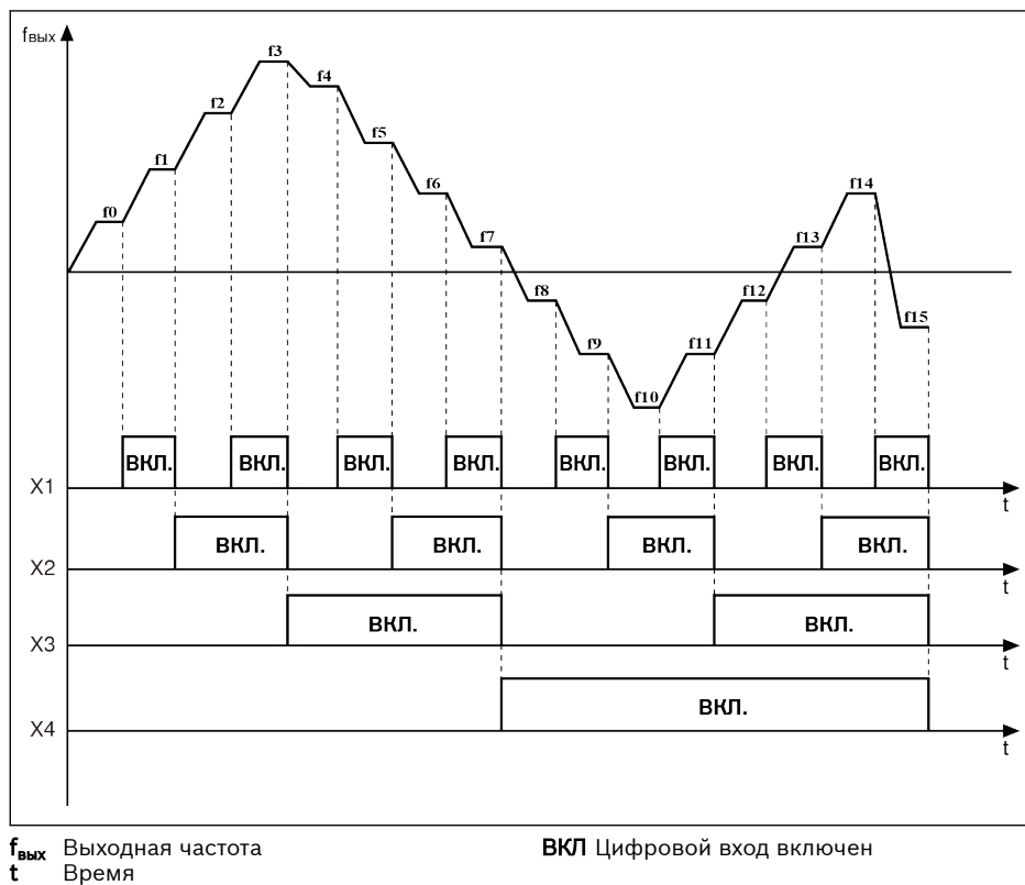
Рис. 12-17: Переход в фазу многоскоростного режима
