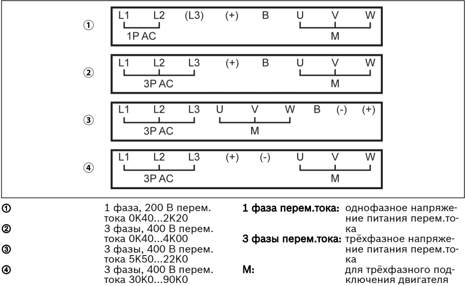
Рис. 8-4: Силовые клеммы
