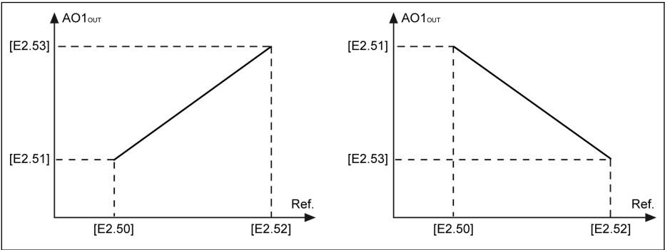
выход AO1 Выход AO1 Опор. Опорное значение Рис. 12-5: Кривая выхода AO1
