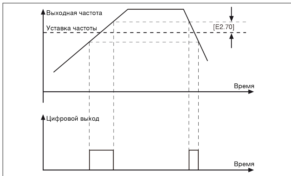
Рис. 12-40: Достижение частоты
