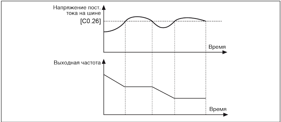
Рис. 12-50: Предотвращение скачков напряжения при торможении
