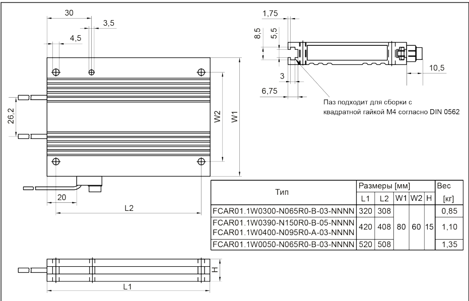
Рис. 15-25: Размеры тормозного резистора_2
