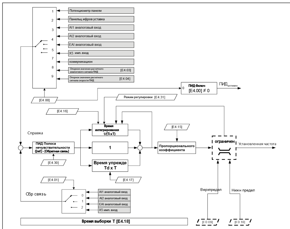
Рис. 12-45: Принцип ПИД-регулирования
