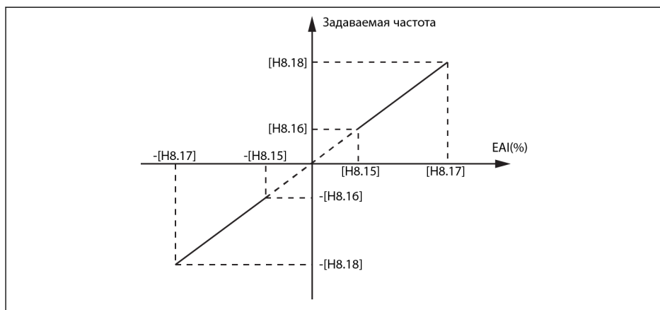
Рис. 12-6: Задание кривой 0
