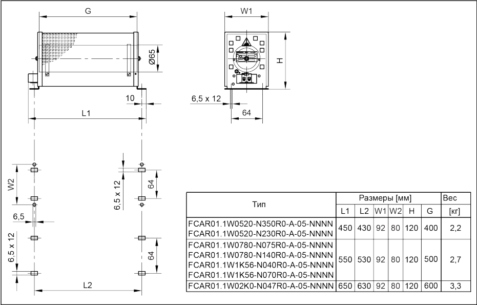
Рис. 15-24: Размеры тормозного резистора_1
