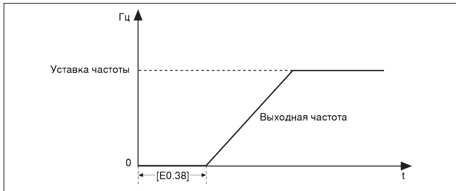
Рис. 12-26: Торможение пост. током перед запуском
