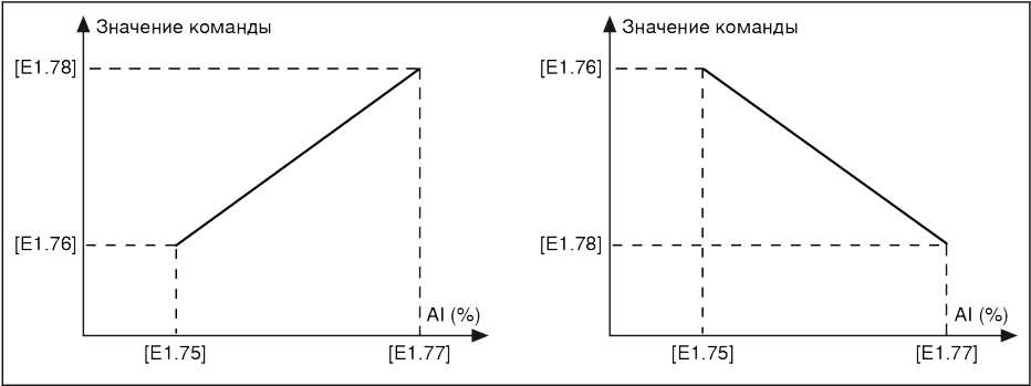
Рис. 12-4: Кривая 2
