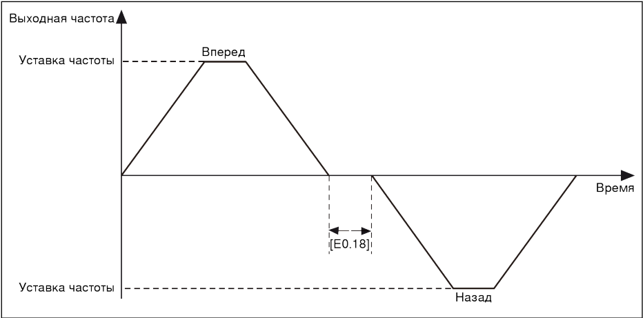
Рис. 12-24: Время задержки смены направления
